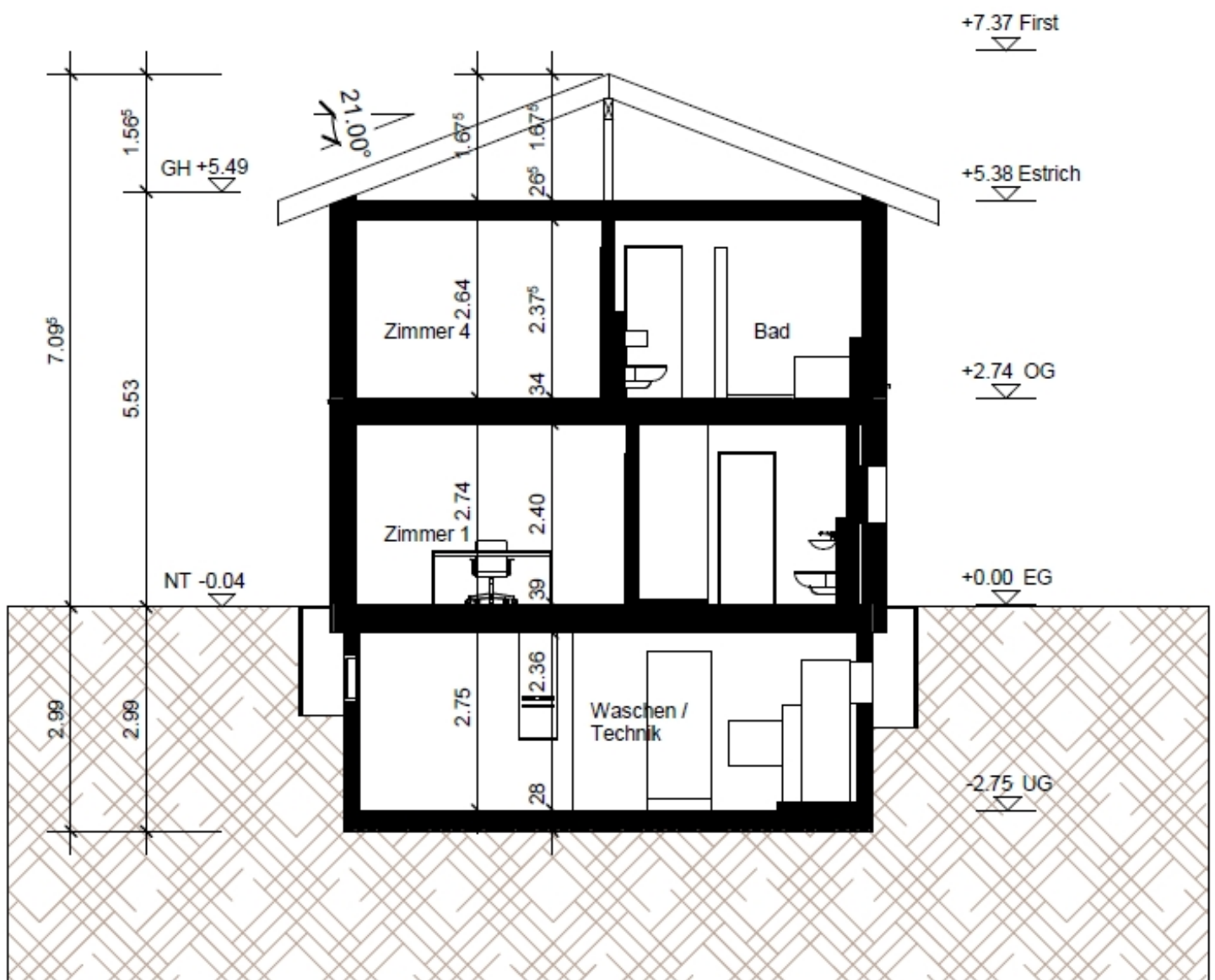
Schnitt
